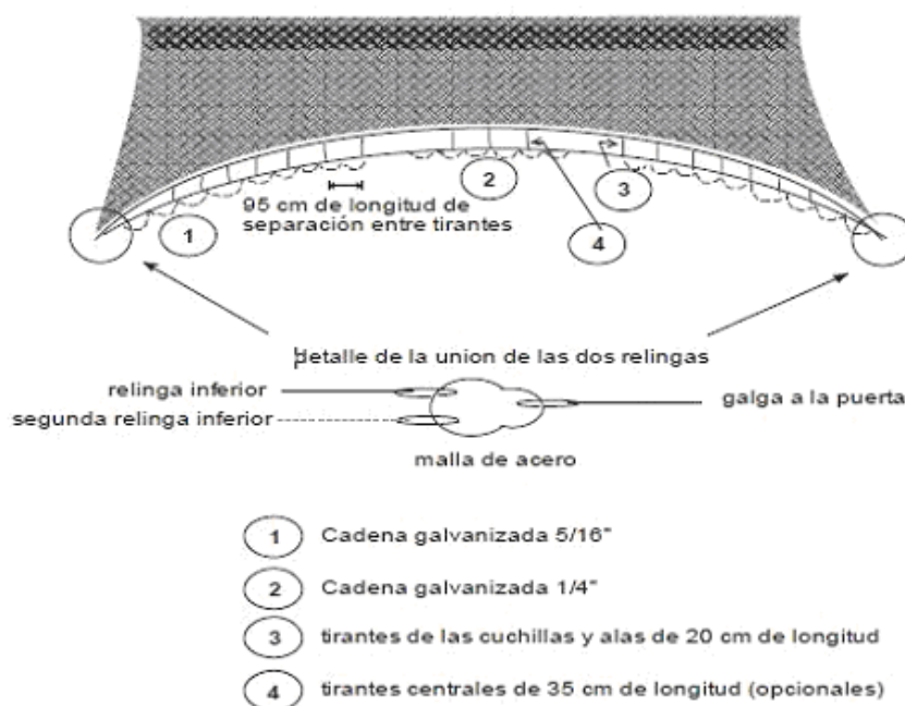
Figura C1. Detalle de armado de la segunda relinga inferior en la red de 33.55 metros (110 pies) para
